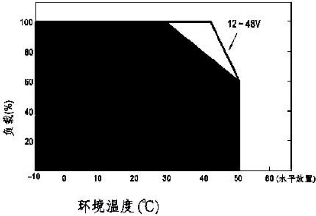
AMBIENT TEMPERATURE(°C)
